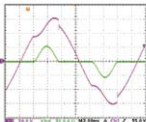
图 3: 实际 RLC 线路
