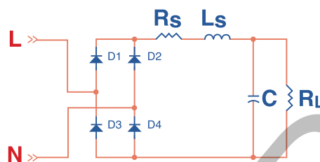
图2: 典型桥式整流线路
