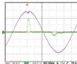
图 6: 浪涌电流模式
